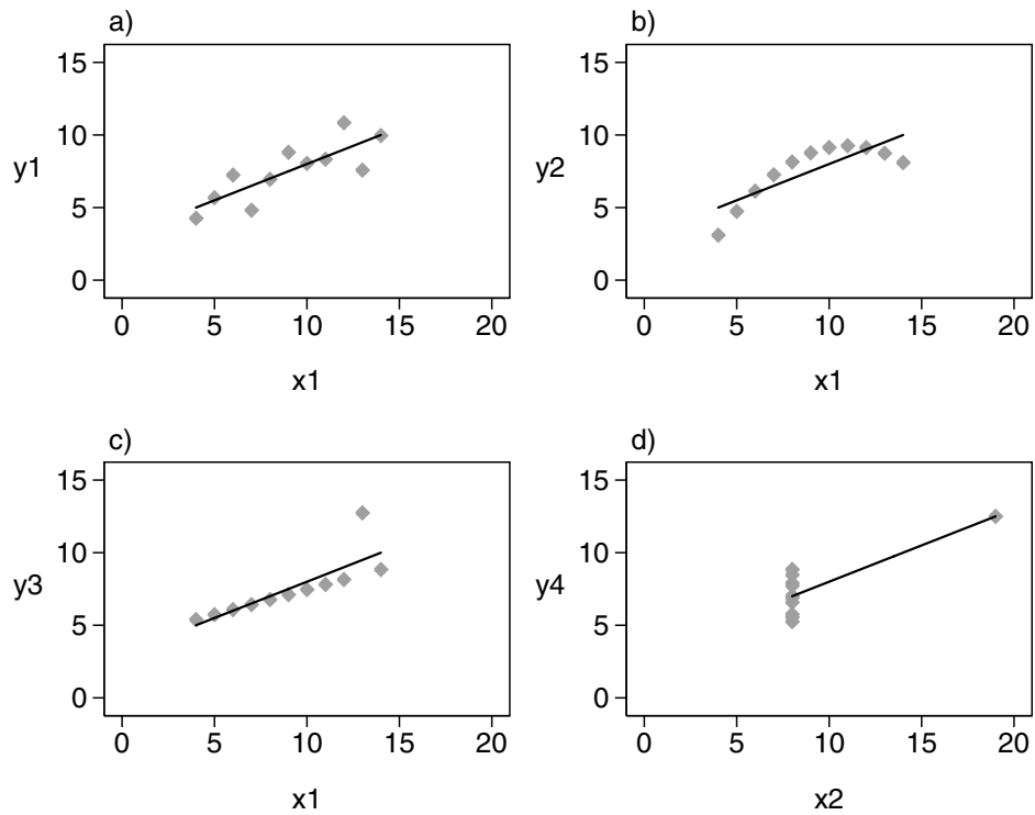
Abbildung 1: Anscombes Quartet
